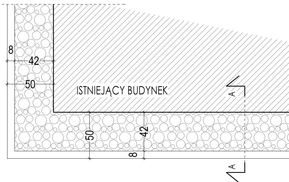
RZUT OPASKI WOKÓŁ BUDYNKU
