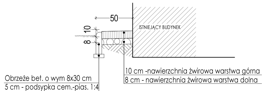
PRZEKRÓJ AA PRZEZ NA WIERZCHNIĘ UTWARDZONA
