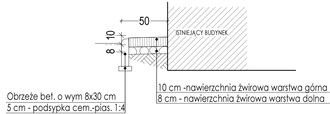
PRZEKRÓJ AA PRZEZ NAWIERZCHNIĘ UTWRADZONA
