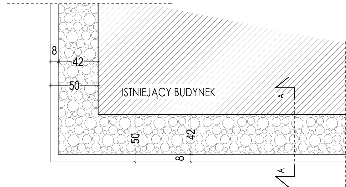
RZUT OPASKI WOKÓŁ BUDYNKU
